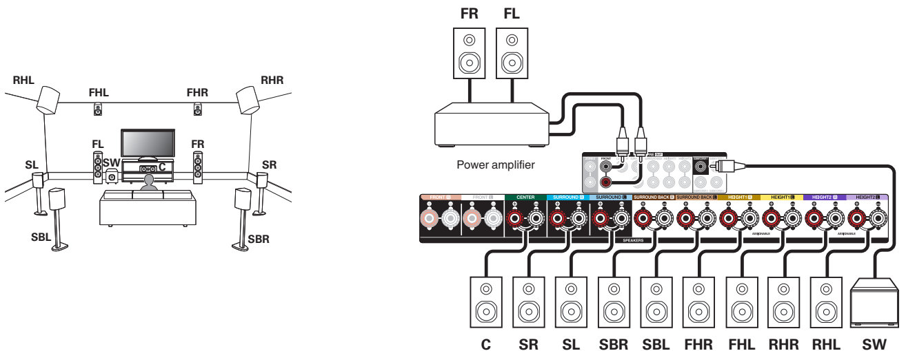
תצורת 11.1 עם רמקולים הקפיים אחוריים ושני זוגות רמקולים גבוהים
