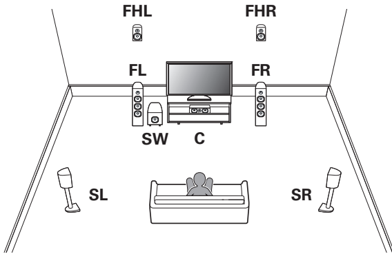
תצורת 7.1 עם רמקולים קדמיים גבוהים
