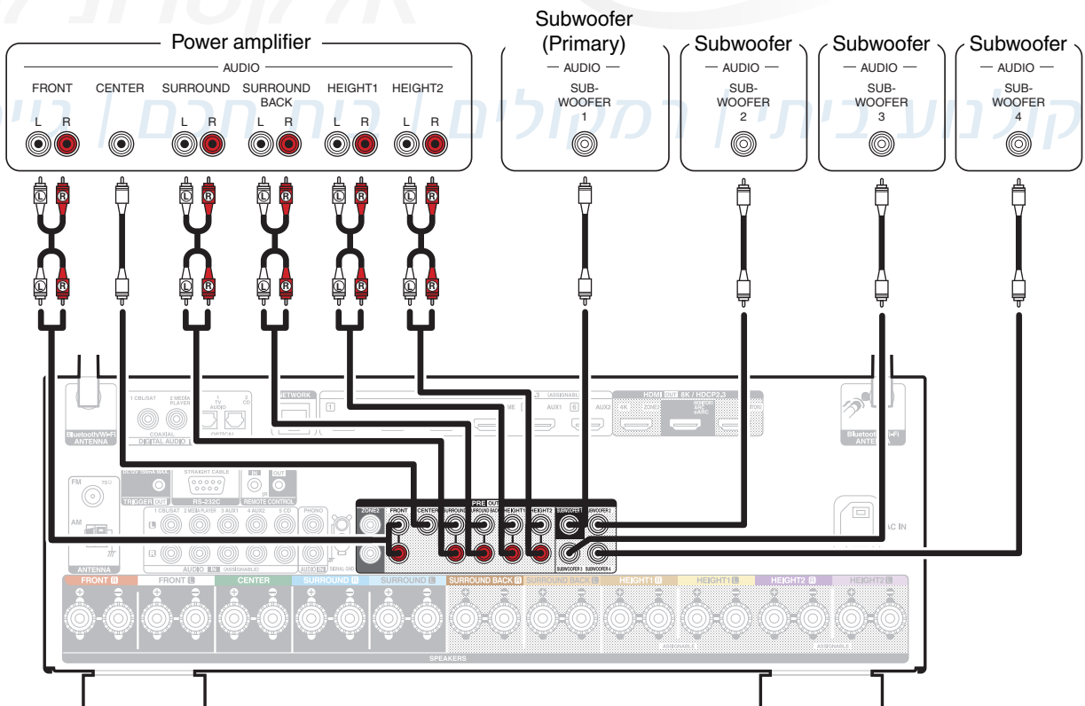
חיבור מגבר חיצוני
