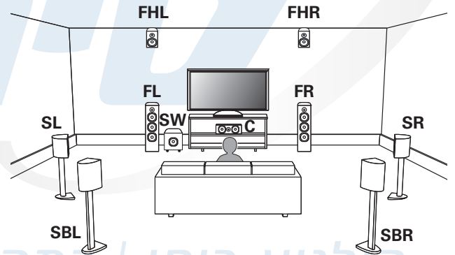
תצורת 9.1 עם רמקולים הקפיים אחוריים וקדמיים גבוהים
