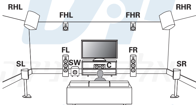
תצורת 9.1 עם שני זוגות רמקולים קדמיים גבוהים
