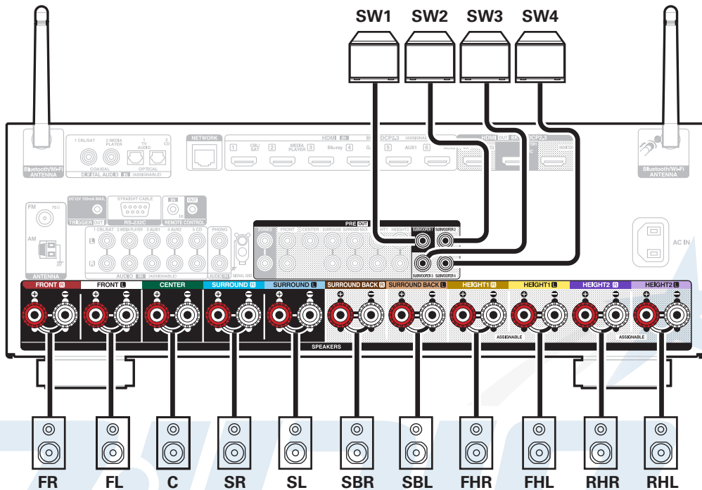
תצורת 11.4 של ברירת מחדל
